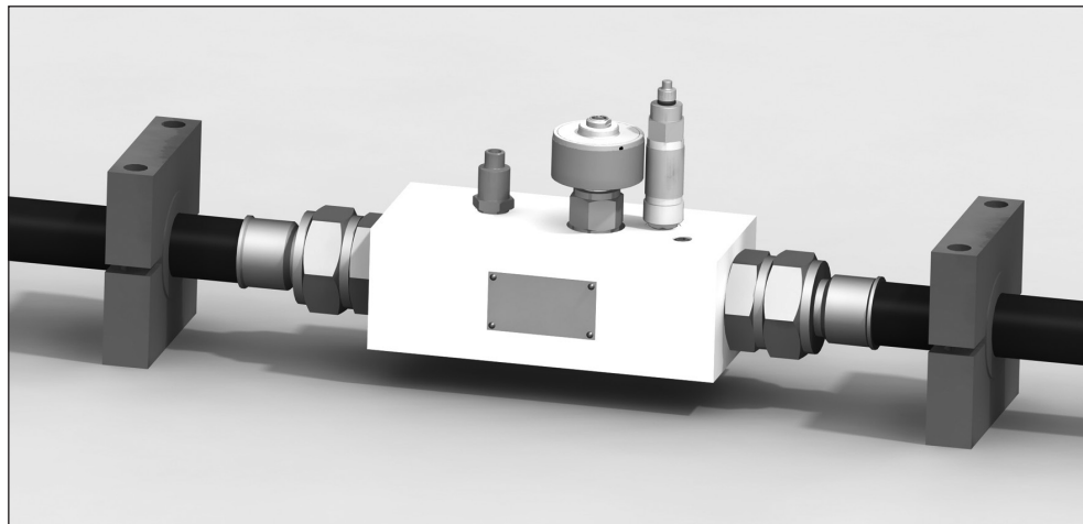
Caudalímetro serie CT con transductores opcionales de temperatura y presión instalados
