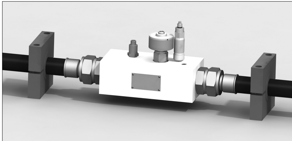
Présentation d'un débitmètre CT avec les options capteur de pression et capteur de température montées.
