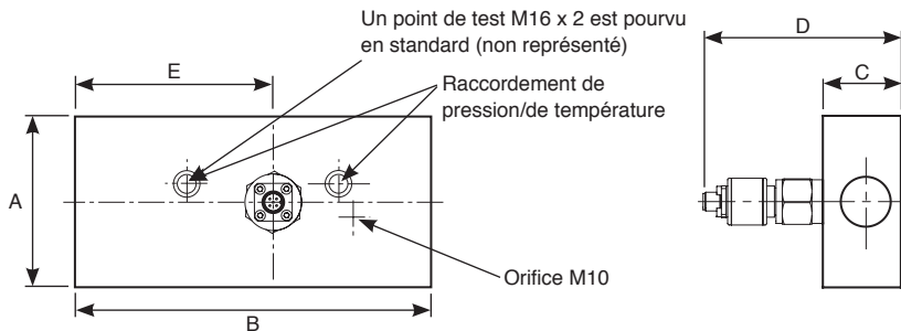
LT15 a un seul orifice pression/température
