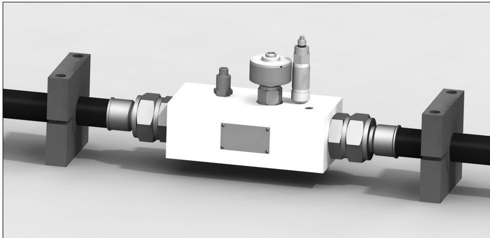
Abb. CT-Durchflussmesser mit montiertem Temperatur- und Druckwandler (Zubehör)
